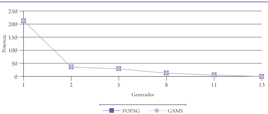
Figura 4. Comparación de potencias en generadores entre Matlab y Gams Power IEEE 30 buses
