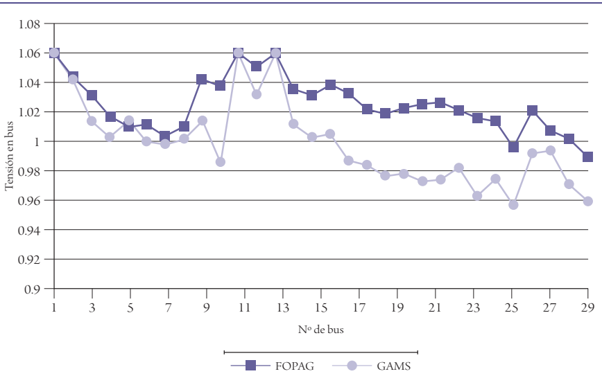
Figura 3. Comparación de tensiones en buses entre Matlab y Gams Power IEEE 30 buses
