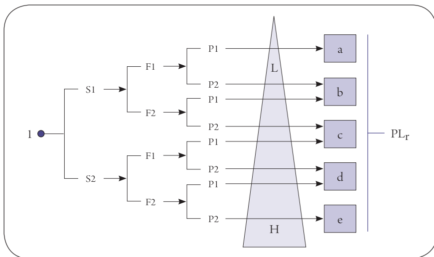
Figura 2. Selección de riesgo y determinación del PLr según la norma EN ISO 13849-1
